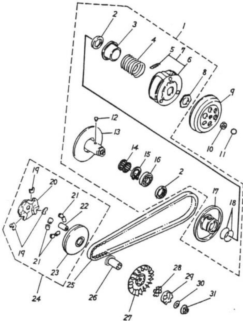
Variomatik 135-10
