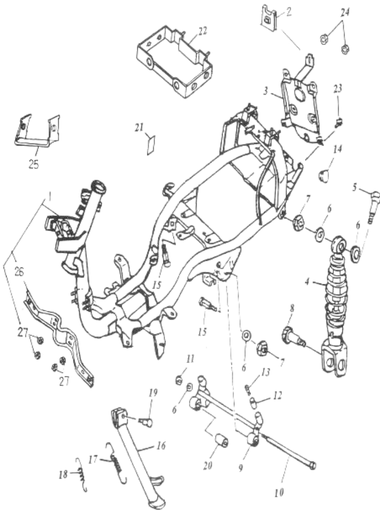
Rahmen 135-13
