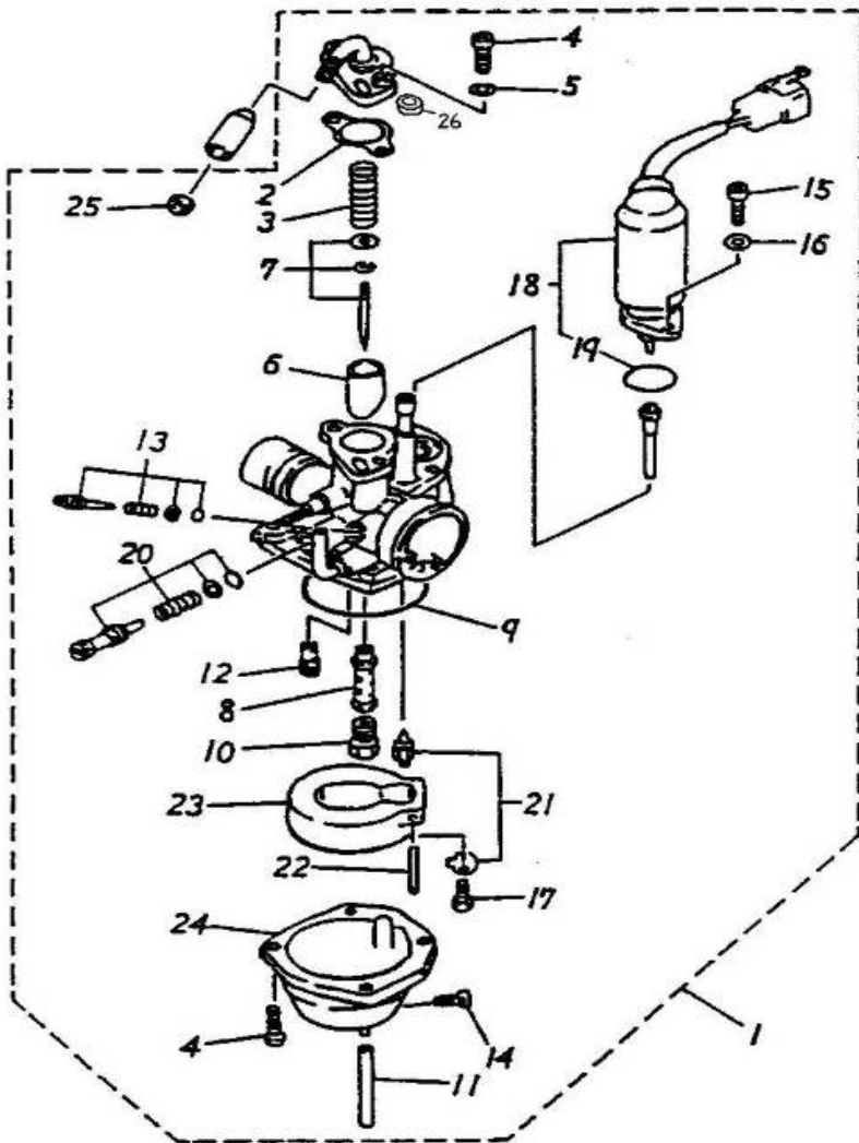
Vergaser 135-06 A
