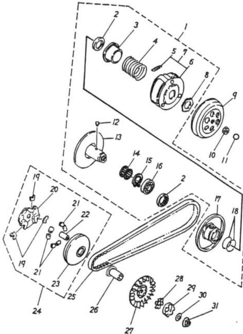
Variomatik 190-10
