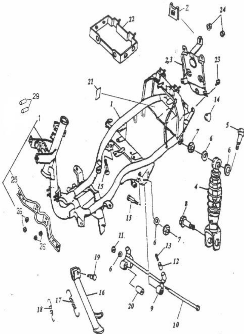
Rahmen 190-13
