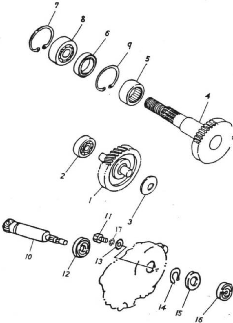
Getriebe 190-11
