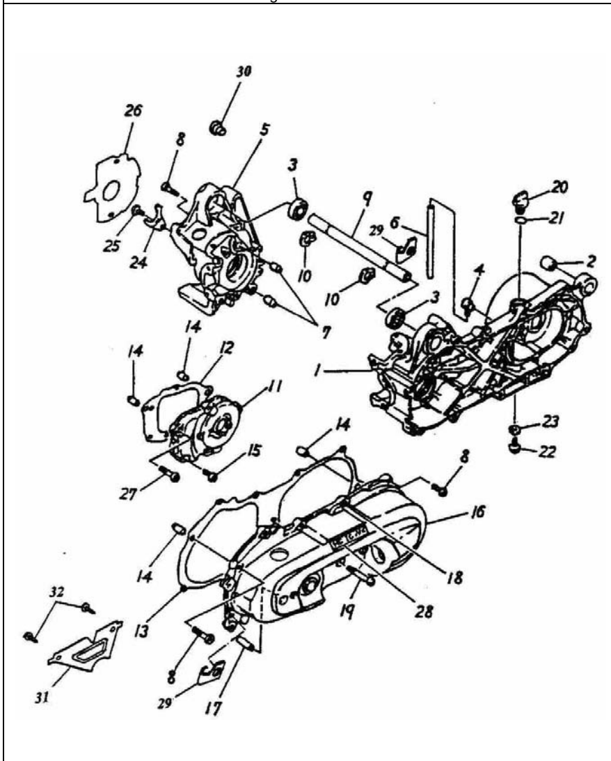
Kurbelgehäuse 1 159-08
