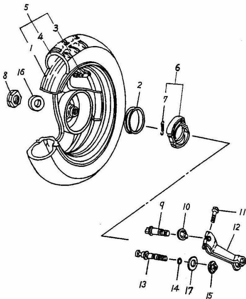
Hinterrad 159-20 A
