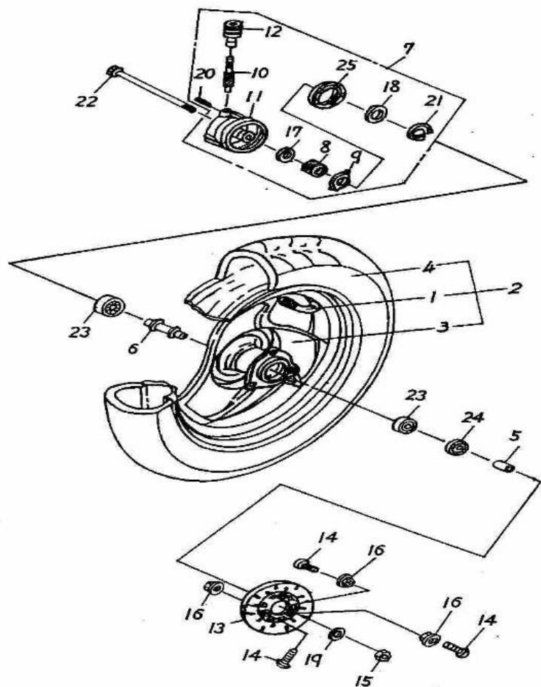
Vorderrad 159-19 A
