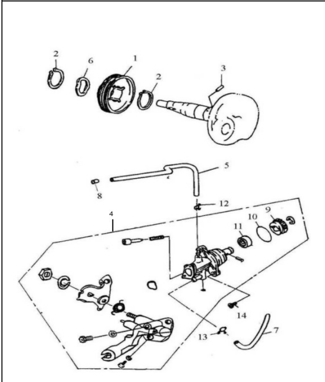
Membrane und Luftfilter 141-05
