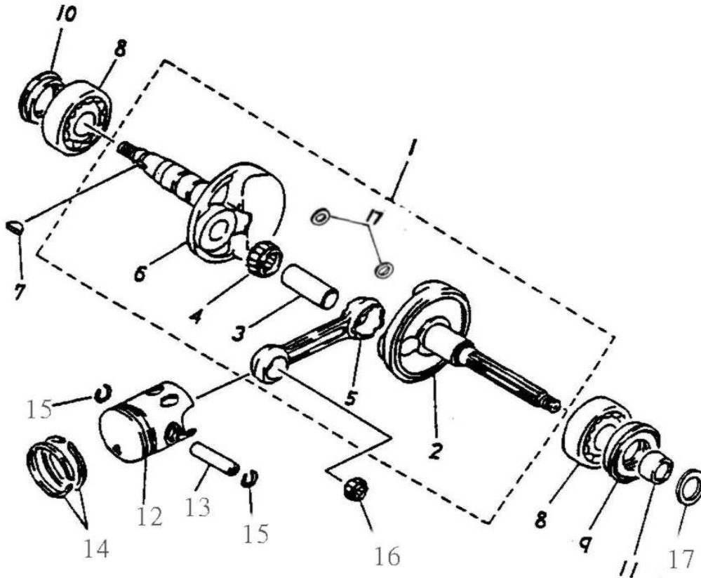
Kurbelwelle 186-02
