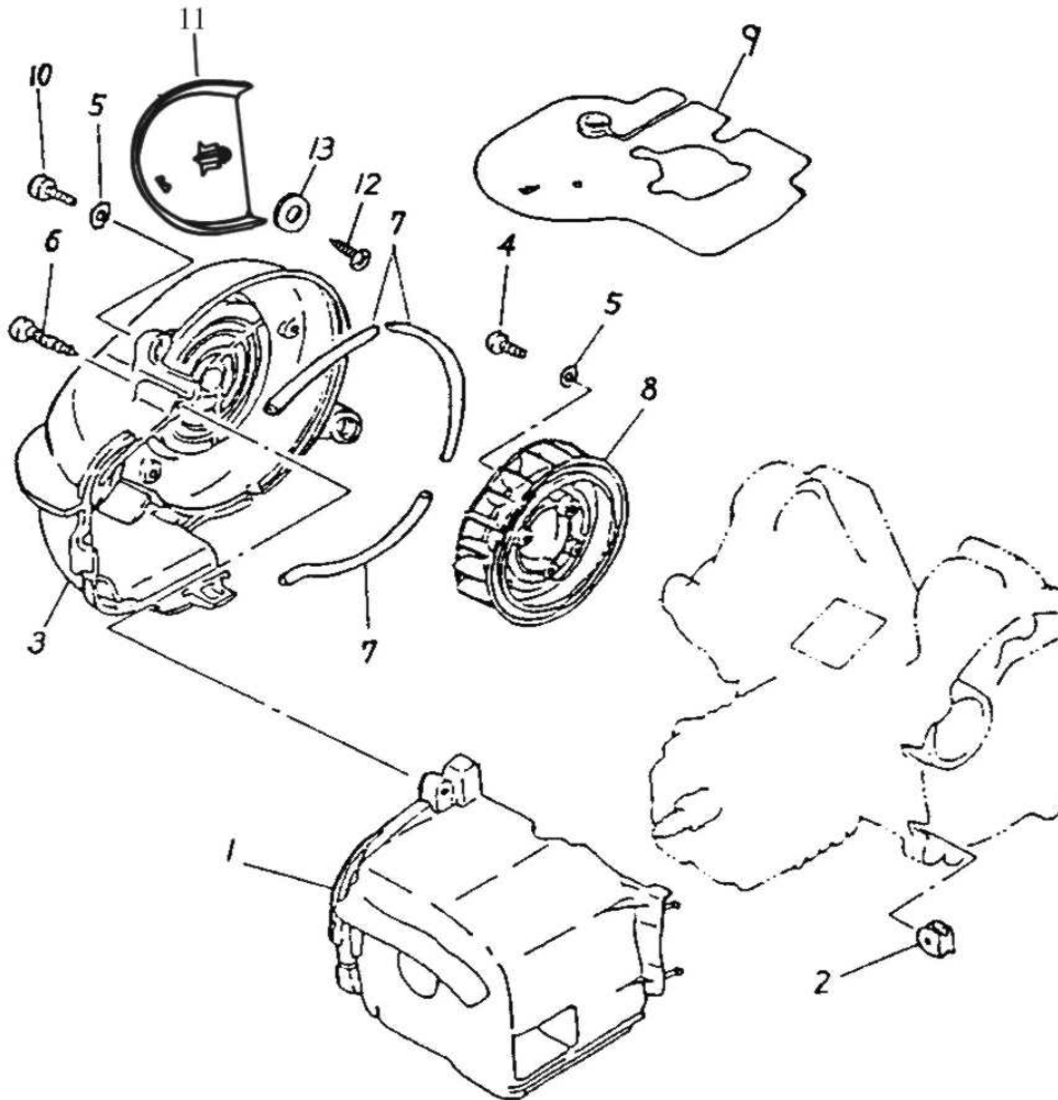
Lüftergehäuse 186-03
