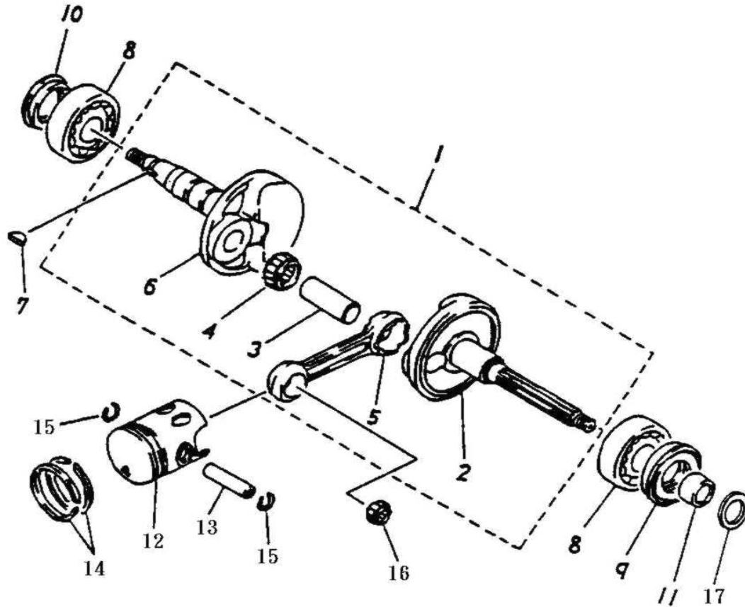
Kurbelwelle 181-02
