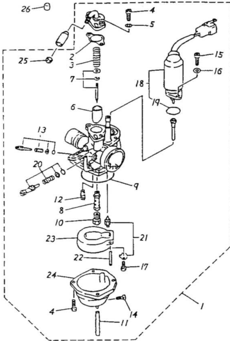
Vergaser 181-06
