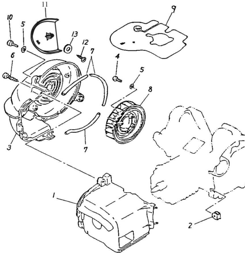
Lüftergehäuse 181-03
